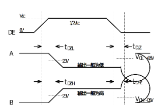
图 6 驱动器使能/关断时序
