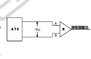
图 9 接收器传输延时测试电
