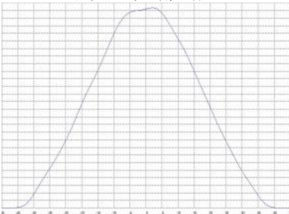
配光曲线-直角坐标
