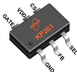
SOT23-6L
