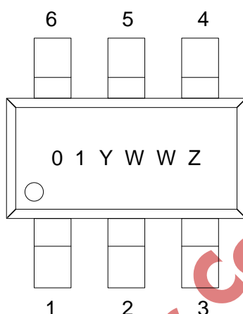
SOT23-6L
