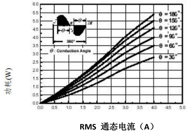
图四、通态电流——最大功耗
