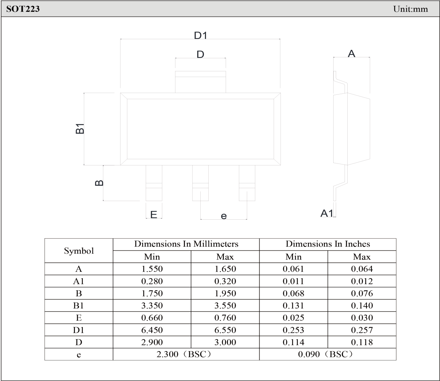
封装外形图:
